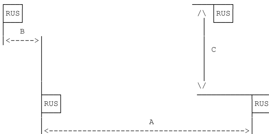
Рис. 1. Фрагмент размещения защитных элементов (А - интервал между элементами в горизонтальном ряду; В - смещение рядов защитных элементов по горизонтали относительно друг друга; С - расстояние между рядами)
